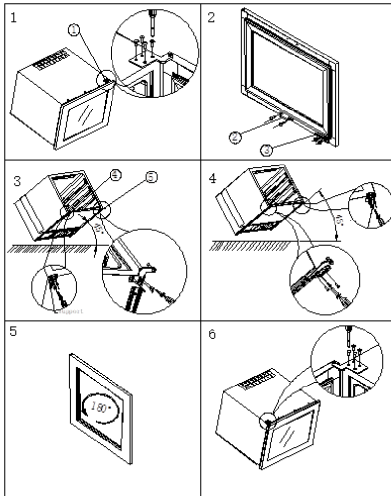
(1) Bovenste scharnier (2) Deur lichtschakelaar (3) Plaatsingsplaat (4) Onderste scharnier (5) Onderste scharnier
