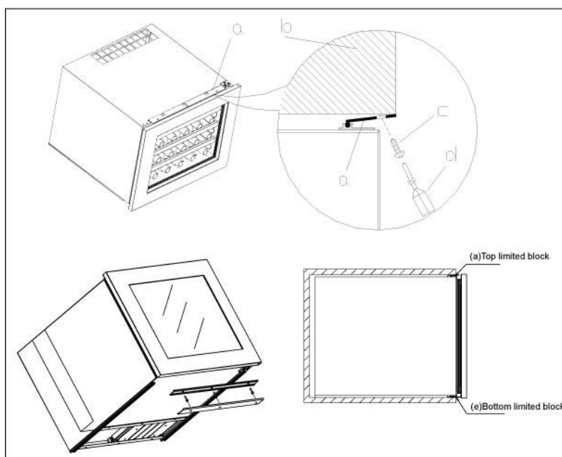
a. Fissaggio superiore b. Frigo cantina c. Viti d. Cacciavite e. Fissaggio inferiore
